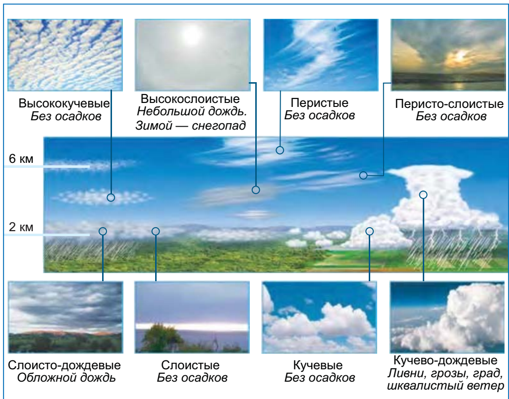
Рис. 98. Типы облаков
