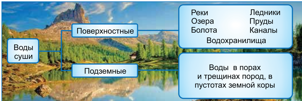
Рис. 94. Воды суши
