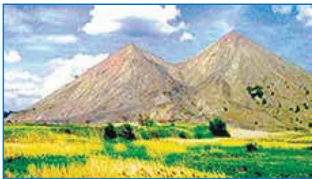
Рис. 64. Терриконы
